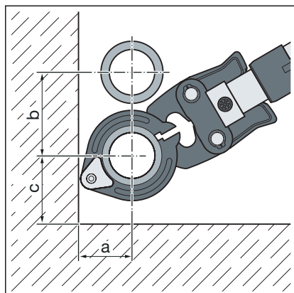
potřebný prostor pro lisovací prstence D 1/2–2
