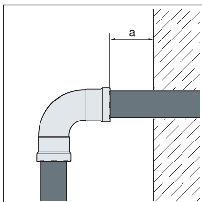
minimální odstup u lisovacích čelistí D 3/4–1
