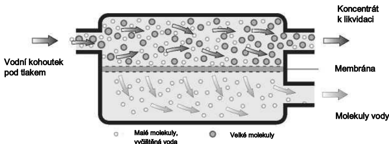
Obr. 1. Zobrazení procesu reverzní osmózy
