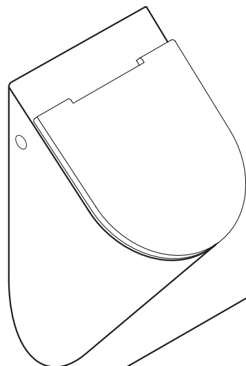
D - Serrare i fissaggi laterali Screw the lateral fixings Seitliche Fixierschrauben festziehen
