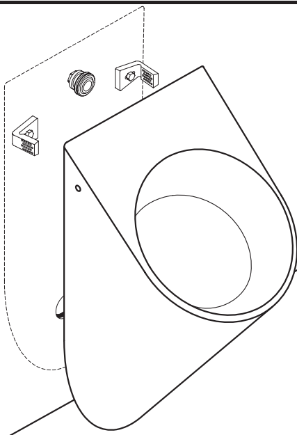
C - Posizionare l'orinatoio a parete Place the urinal back to wall Urinal an der Wand positionieren
