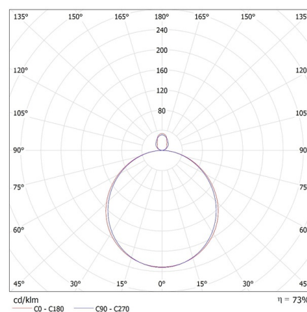
MILED0 (kat 31510) AZPO LED 22W-NW-L-W / Krzywa rozsyłu światła (biegunowo)
