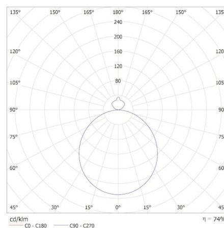
MILED0 (kat 31506) AZPO LED 12,3W-NW-L-W / Krzywa rozsyłu światła (biegunowo)
