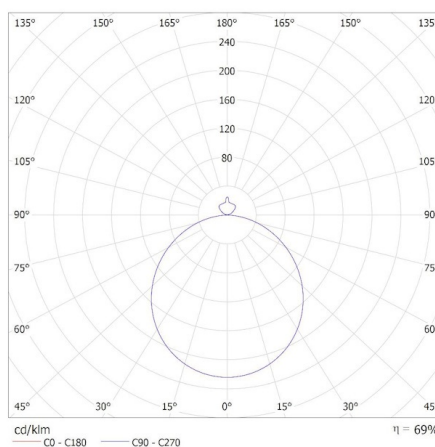
MILED o (kat 31500) AZPO LED 11,8W-NW-O-W / Krzywa rozsyłu światła (biegunowo)
