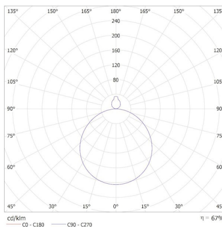
MILED0 (kat 31503) AZPO LED 18,5W-NW-O-B / Krzywa rozsyłu światła (biegunowo)
