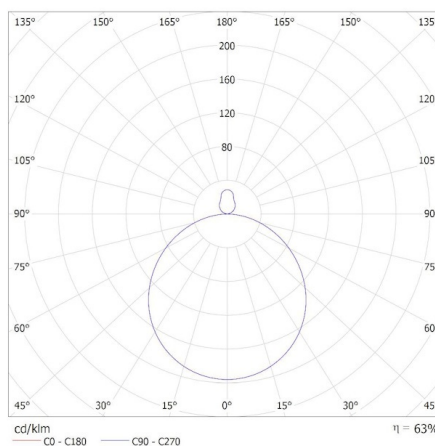
MILEDO (kat 31504) AZPO LED 22W-NW-O-W / Krzywa rozsyłu światła (biegunowo)
