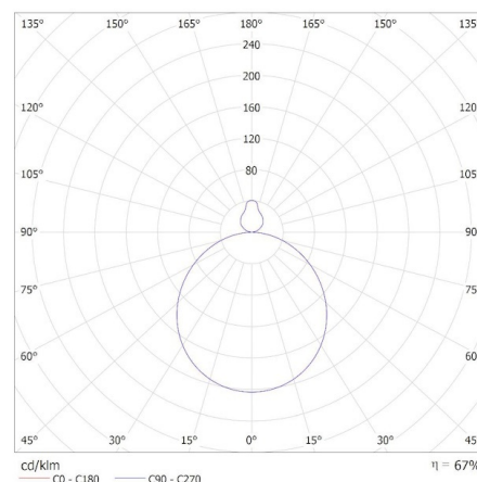
MILED (kat 31509) AZPO LED 17,5W-NW-L-B / Krzywa rozsyłu światła (biegunowo)
